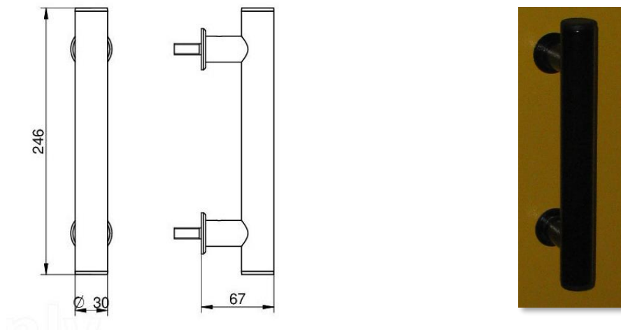
Obrázek 7 Madlo pro ŠD VDLM - U
