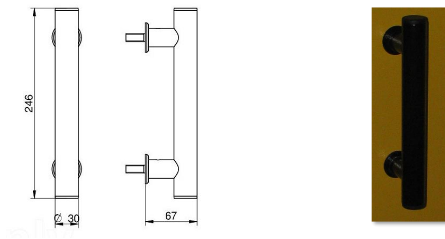
Obrázek 14 Madlo pro ŠD VDLM - D
