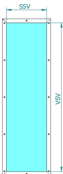
Obrázek 15 Rámeček prosklení a skleněná výplň ŠD VDLM - D
