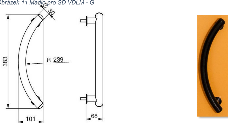
Obrázek 11 Madlo pro ŠD VDLM - G
